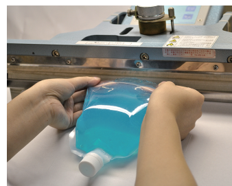
シールによる密封
